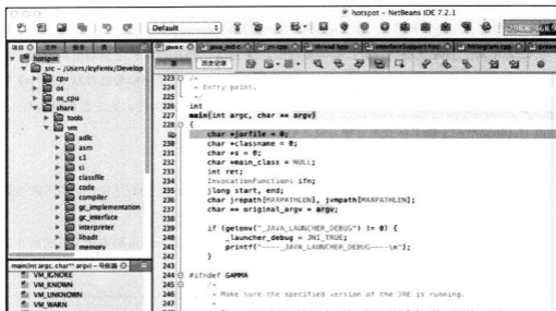
图 1-11 在 NetBeans 中创建 HotSpot 项目 (4)
