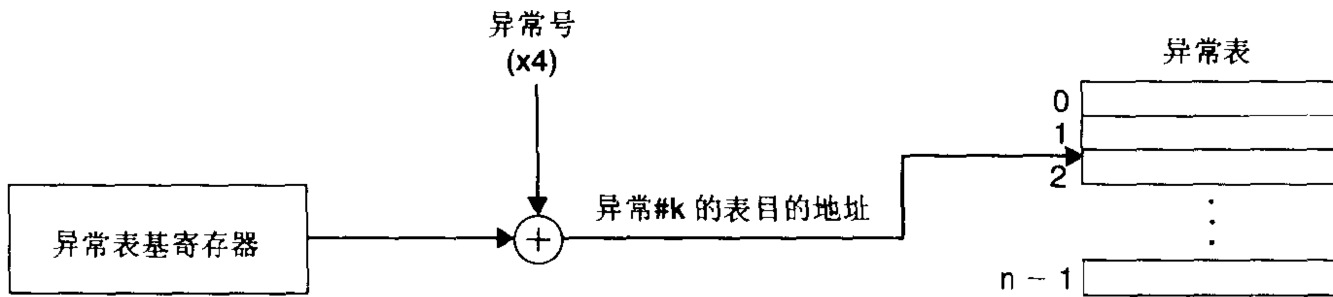
图 8.3 生成异常处理程序的地址
