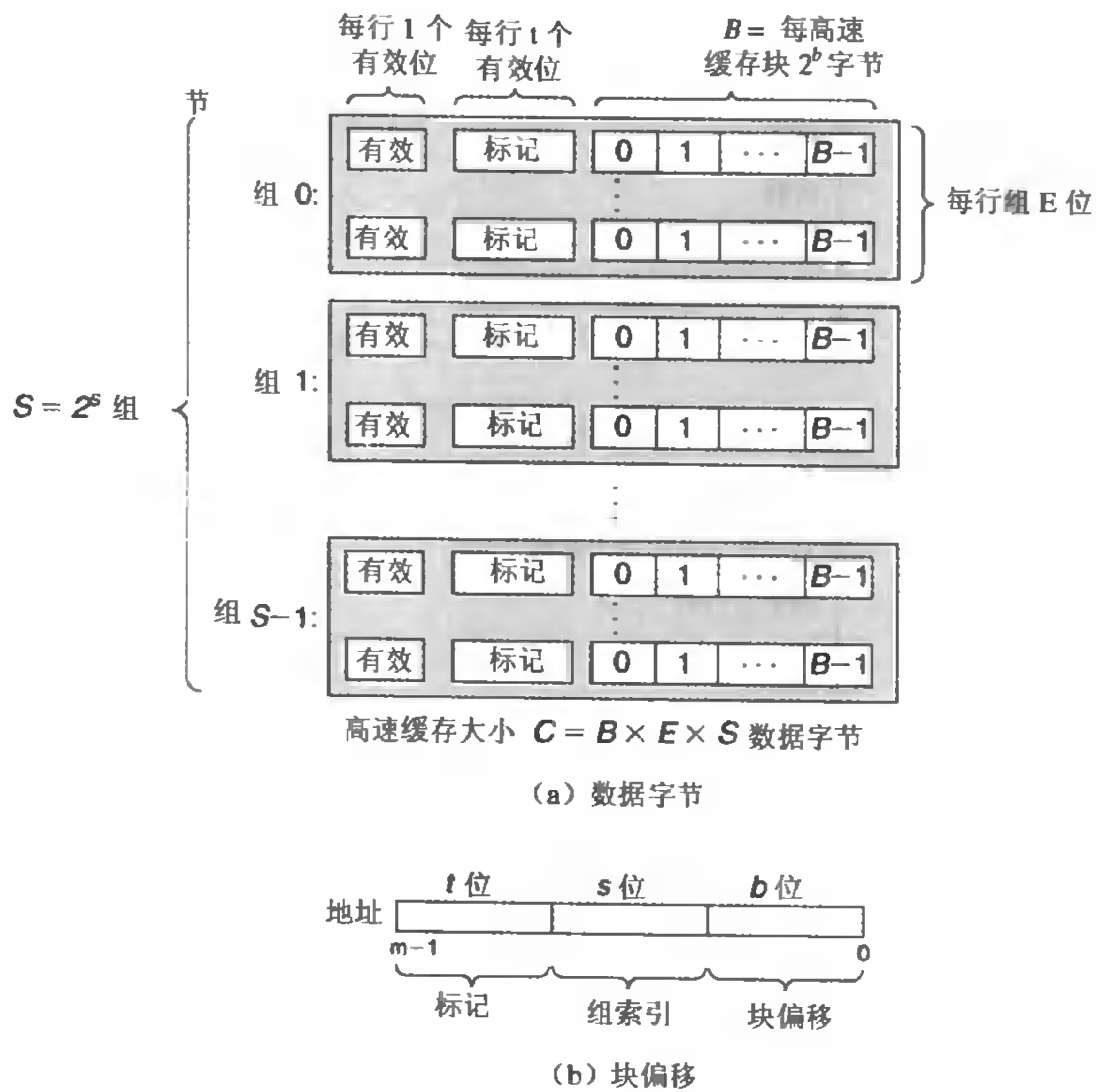
图 6.25 高速缓存 (S,E,B,m) 的通用结构
