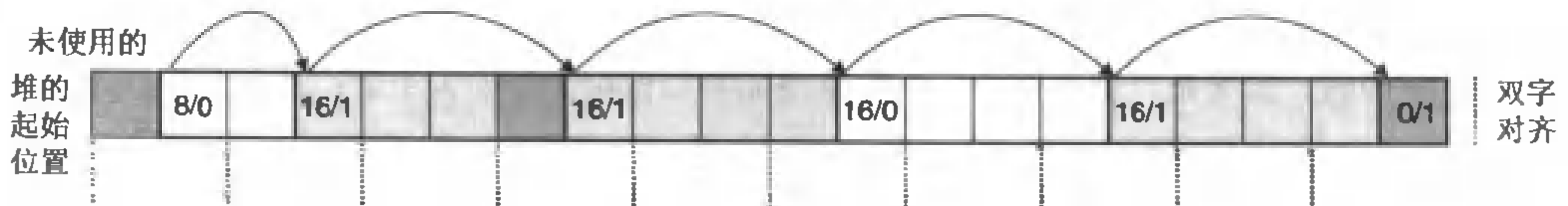
图 10.39 分割一个空闲块，以满足一个 3 个字的分配请求
