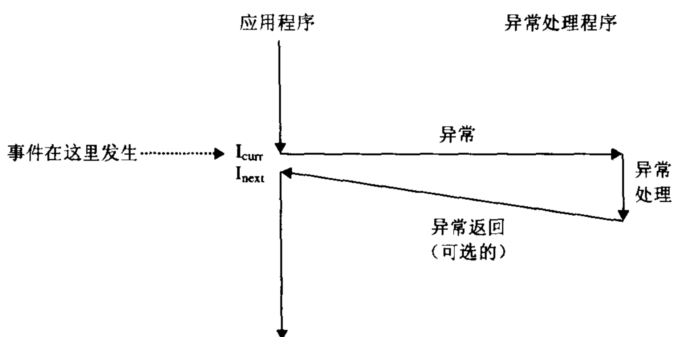
图 8.1 异常的剖析
