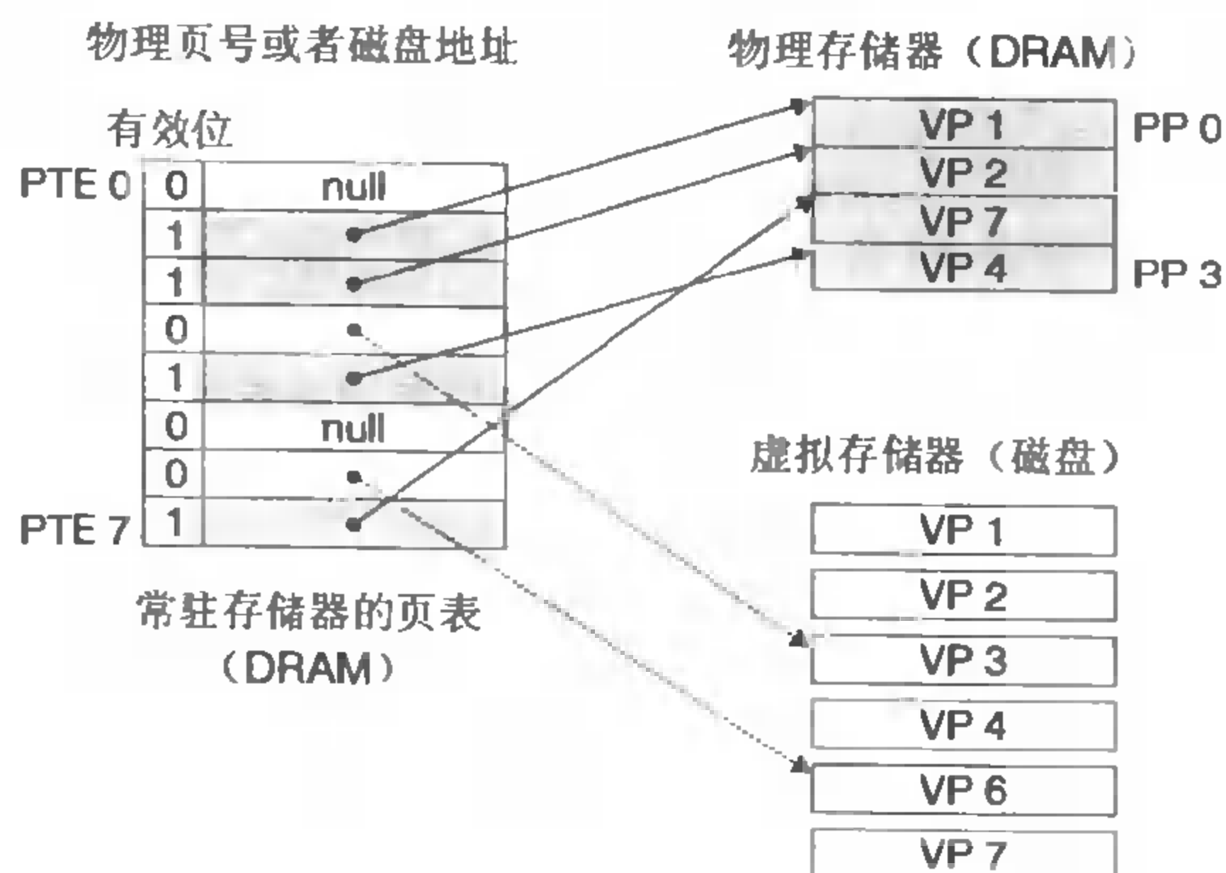
图 10.4 页表
