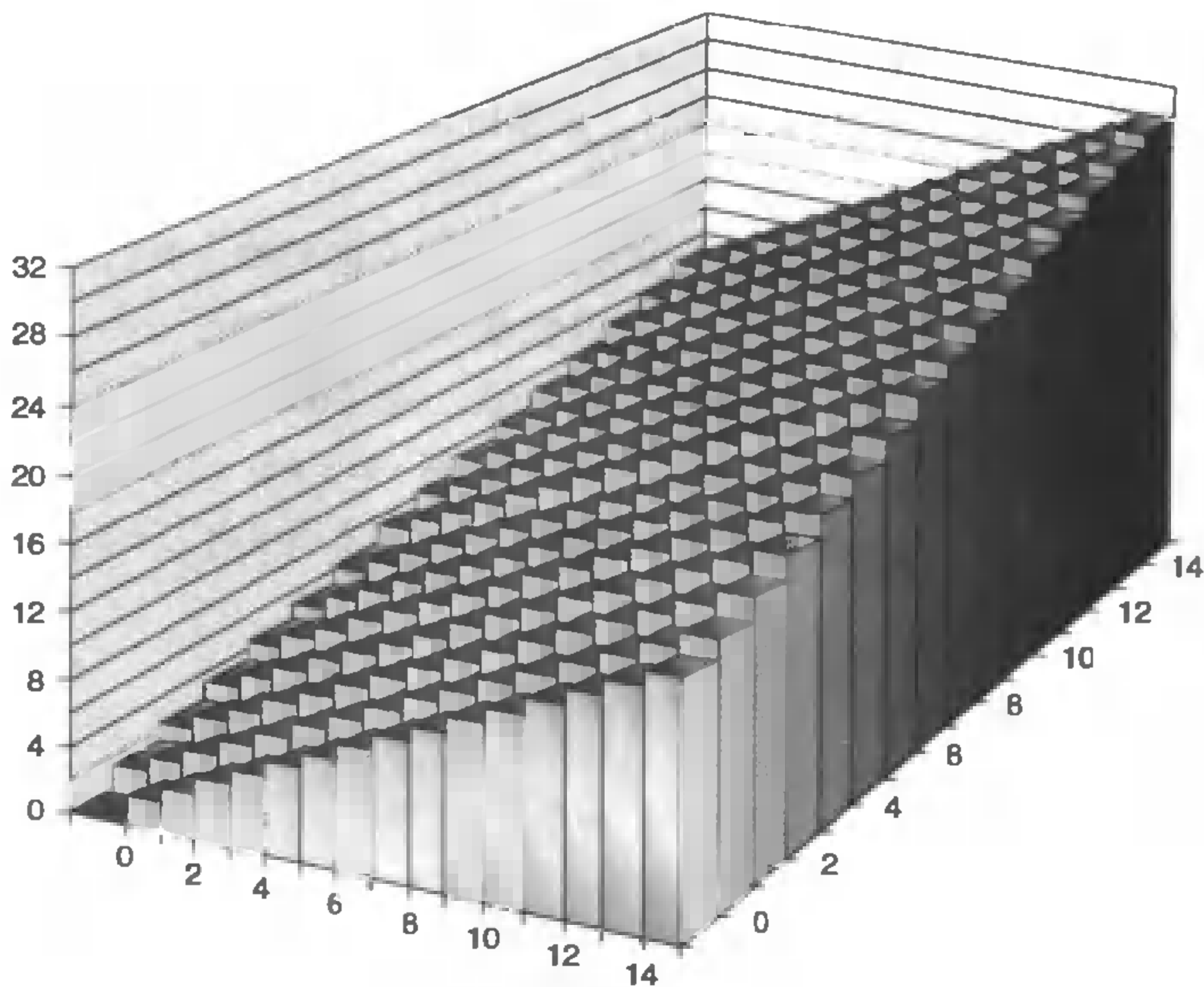
图 2.14 整数加法
