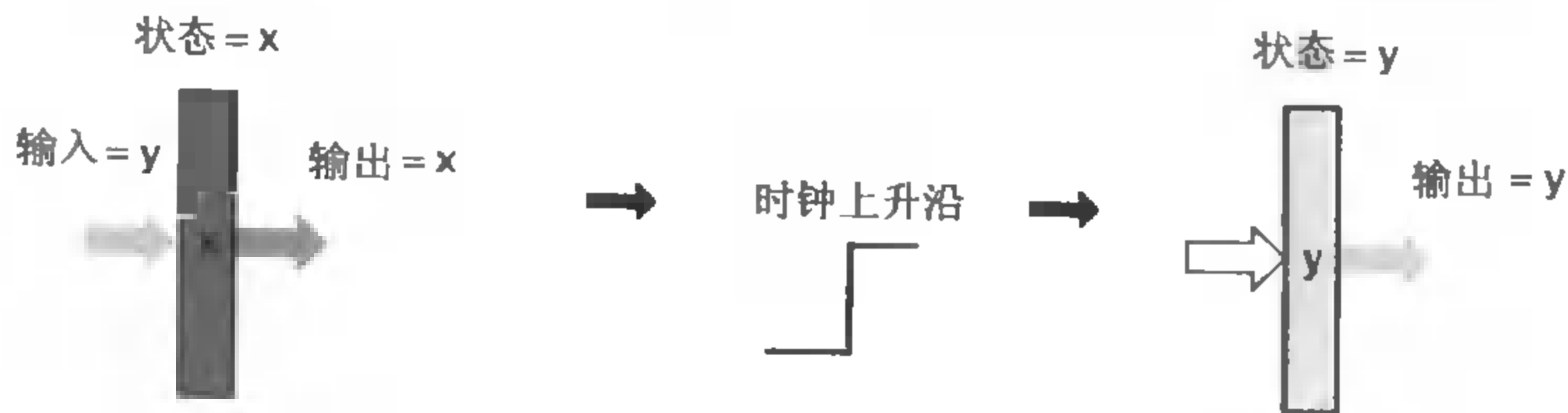
图 4.14 寄存器操作
